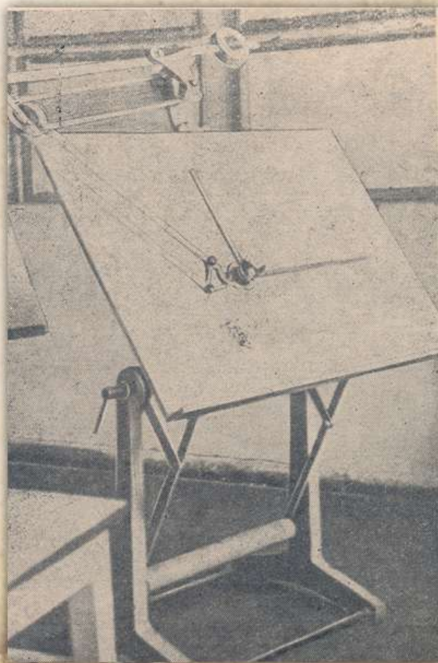
Чертежный прибор – продукция учебно-производственных мастерских, 1960-е гг. Р-605, оп.1, д.23, л.8
